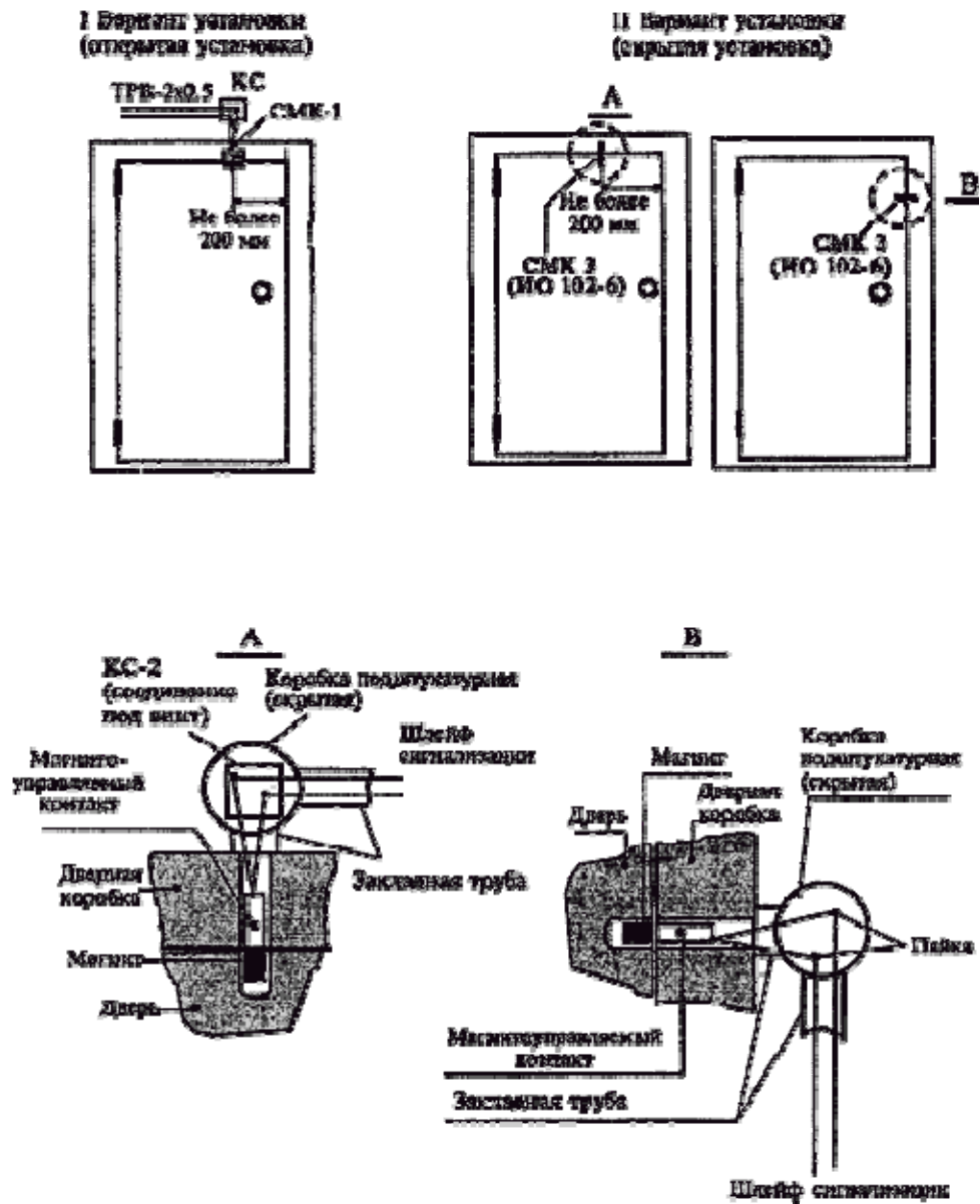
Рисунок 1 - Варианты установки магнитоконтактных извещателей на дверь
