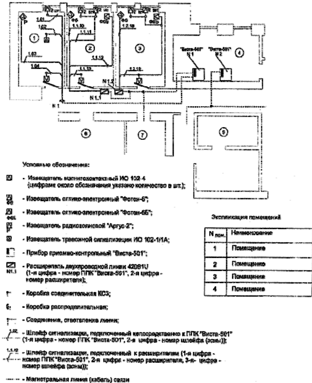
Рисунок 6 - Вариант выполнения схемы плана сети охранной сигнализации на базе ППК "Виста-501"
