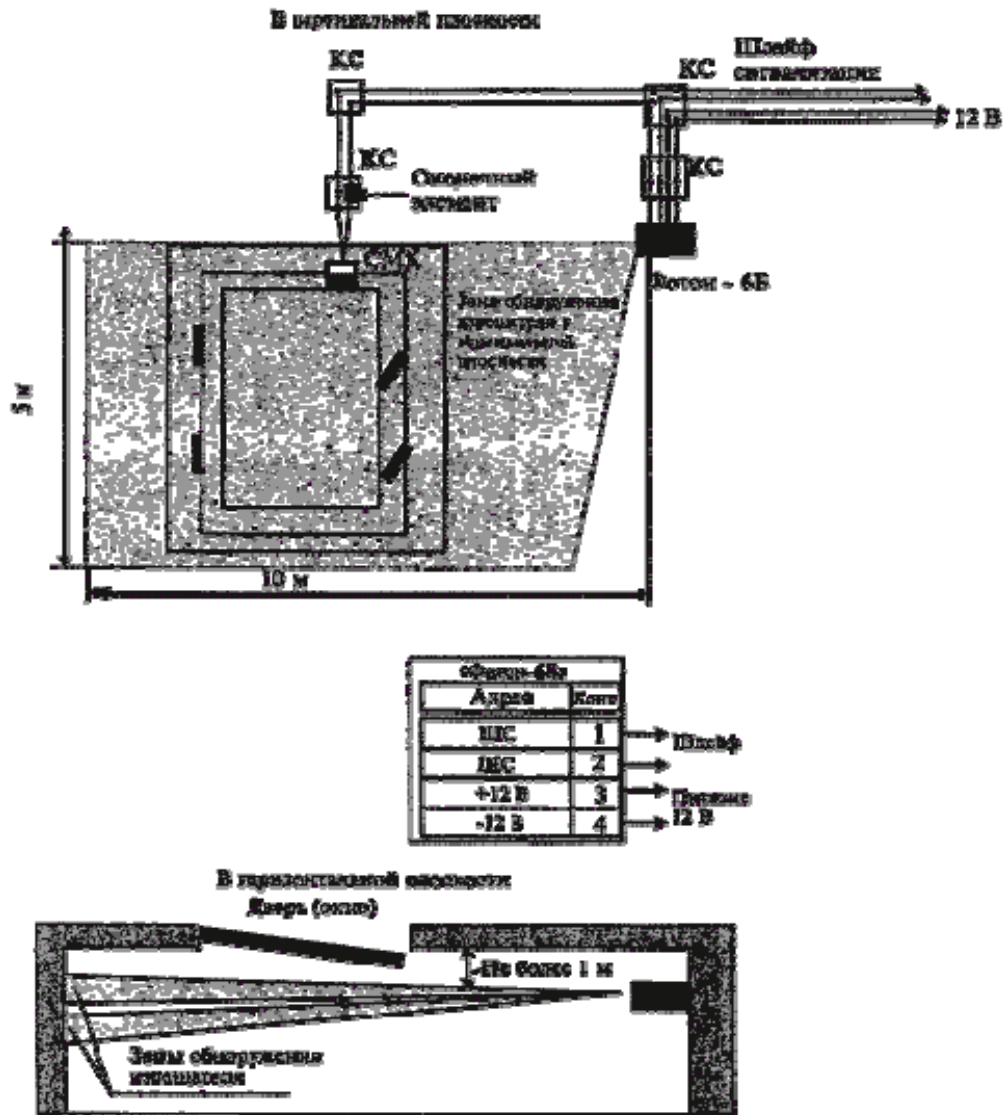
Рисунок 2 - Вариант блокировки двери (окна) на открывание и проникновение. (Размещение и схема подключения извещателей)
