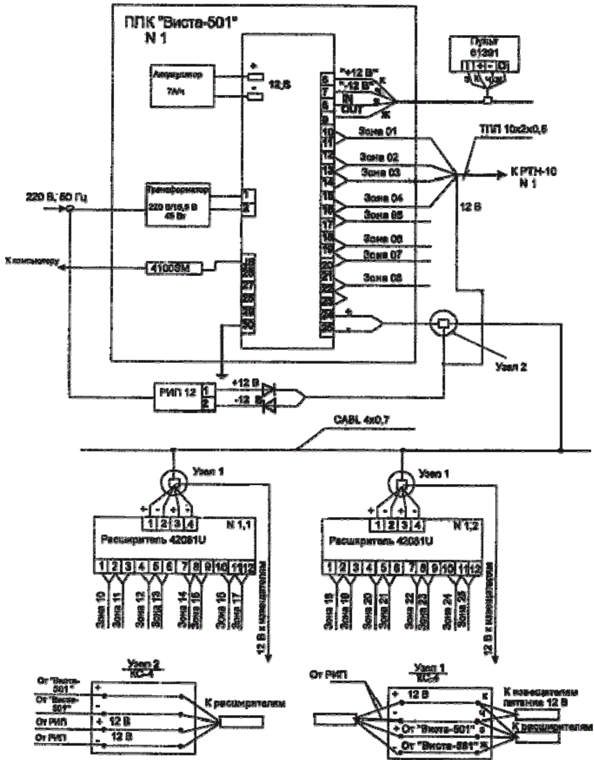
Рисунок 8 - Вариант выполнения электрической схемы соединений 6.4 Схемы соединений структурная и электрическая
