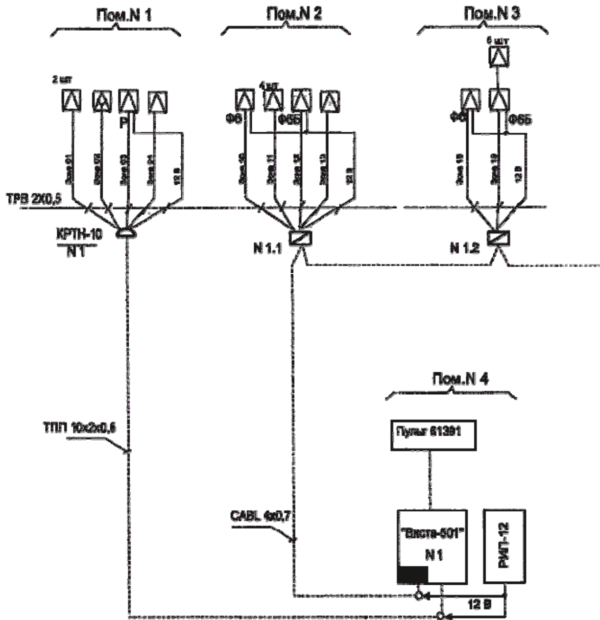
Рисунок 7 - Вариант выполнения структурной схемы соединений
