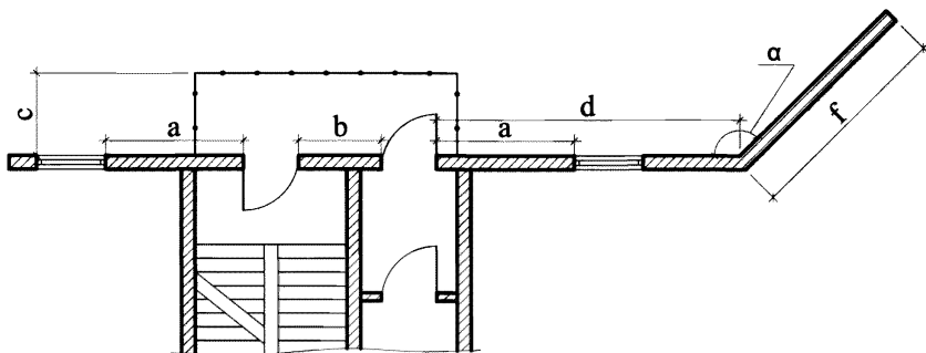
Рисунок 36 – Поэтажные переходы через наружную воздушную зону к незадымляемым лестничным клеткам типа Н1 по балконам с торцевыми сплошными
