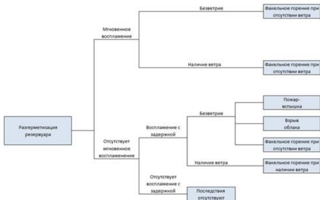
Рис. 3.7.2. Дерево событий при возникновении и развитии пожароопасной ситуации, связанной с разгерметизацией абсорберов 1 и 2 УРУ с парами ЛВЖ
