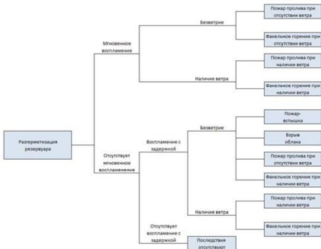
Рис. 3.7.3. Дерево событий при возникновении и развитии пожароопасной ситуации, связанной с разгерметизацией абсорбера 3 и сепаратора УРУ с ЛВЖ, а также трубопроводов налива, технологических трубопроводов и центробежного насоса УРУ
