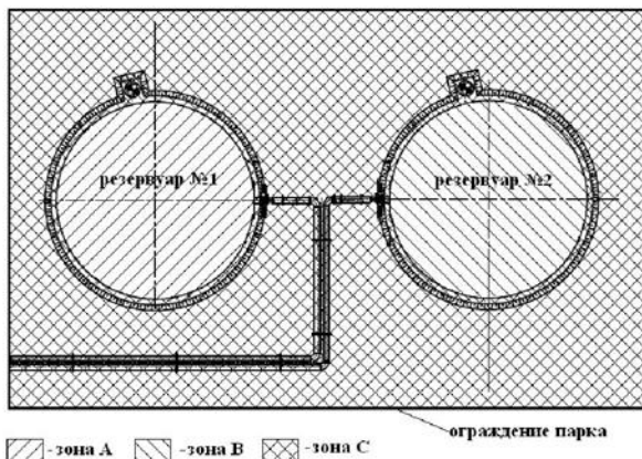
Рис. 3.2.12. Схема резервуаров парка к расчету потенциального пожарного риска в границах обвалования (ограждения)
