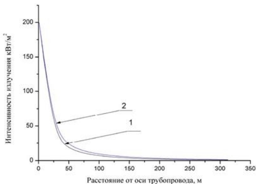
Рис. 3.5.2. Зависимость интенсивности теплового излучения факельного горения от расстояния от оси трубопровода для различных типов повреждений рассматриваемого продуктопровода 1 – «свищ»; 2 – «трещина», «гилютинный разрыв»
