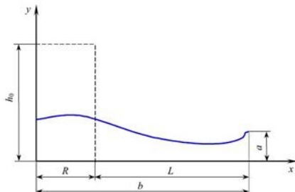
Рис. П4.2. Типичная картина движения жидкости в обваловании при квазимгновенном разрушении резервуара:
