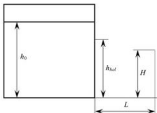
Рис. П.4.1. Схема для расчета истечения жидкости из отверстия в резервуаре
