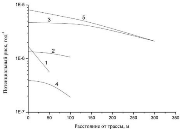
Рис. 3.8.2. Зависимость потенциального пожарного риска от расстояния до трассы для различных сценариев аварии. 1 – факельное горение; 2 – пожар – вспышка при полном разрушении автомобильной цистерны; 3 – огненный шар; 4 – пожар – вспышка при истечении из отверстия диаметром 50 мм; 5 – суммарный потенциальный пожарный риск
