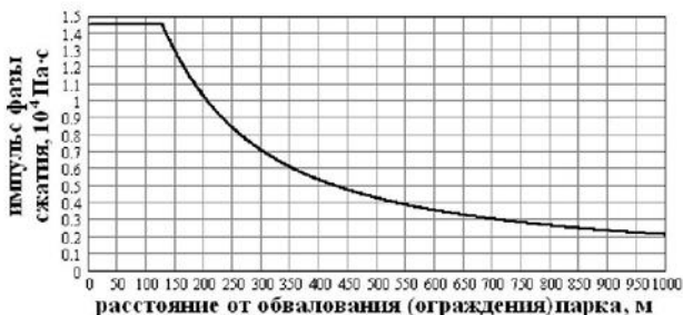
Рис. 3.2.9. Зависимость импульса фазы сжатия в волне давления от расстояния до обвалования (ограждения) парка (масса паров 114700 кг)
