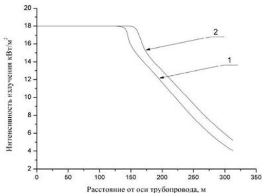
Рис. 3.5.3. Зависимость интенсивности теплового излучения пожара пролива от расстояния от оси трубопровода для различных типов повреждений рассматриваемого продуктопровода 1 – «свищ»; 2 – «трещина», «гилютинный разрыв»
