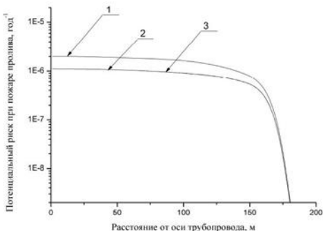
Рис. 3.5.4. Зависимость потенциального пожарного риска пожара пролива от расстояния от оси трубопровода для различных типов повреждений рассматриваемого продуктопровода 1 – «свищ»; 2 – «трещина»; 3 – «гилютинный разрыв»
