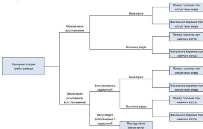
Рис. 3.5.1. Дерево событий развития пожароопасных ситуаций на продуктопроводе
