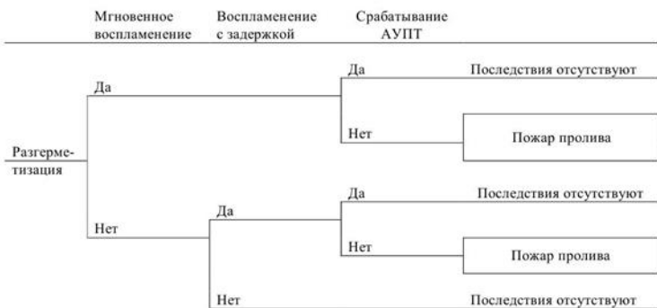
Рис. 3.6.1 Дерево событий для сценариев возникновения и развития пожароопасных ситуаций и пожаров, связанных с разгерметизацией технологического оборудования и поступлением горючих жидкостей в объем помещения
