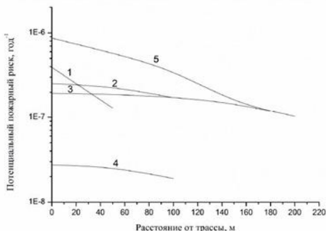
Рис. 3.9.2. Зависимость потенциального пожарного риска от расстояния до трассы прохождения железнодорожного состава с СУГ для различных сценариев аварии. 1 – факельное горение; 2 – пожар – вспышка при полном разрушении железнодорожной вагона-цистерны; 3 – огненный шар; 4 – пожар – вспышка при истечении из отверстия диаметром 50 мм; 5 – суммарный потенциальный пожарный риск
