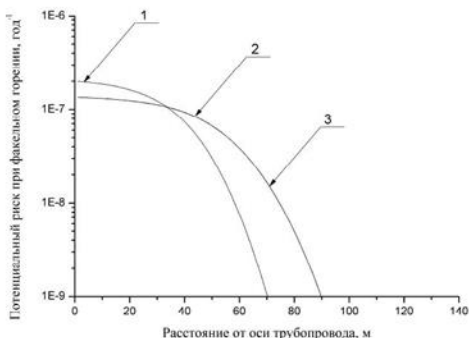
Рис. 3.5.5. Зависимость потенциального пожарного риска факельного горения от расстояния от оси трубопровода для различных типов поврежденный рассматриваемого продуктопровода 1 – «свищ»; 2 – «трещина»; 3 – «гилютинный разрыв»
