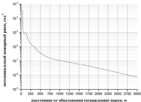
Рис. 3.2.13. Зависимость потенциального пожарного риска от расстояния до обвалования (ограждения) парка
