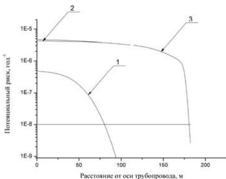
Рис. 3.5.6. Зависимость потенциального пожарного риска от расстояния от оси трубопровода и вклад k-го сценария аварии в величину суммарного потенциального пожарного риска на участке перехода рассматриваемого продуктопровода через водную преграду.
