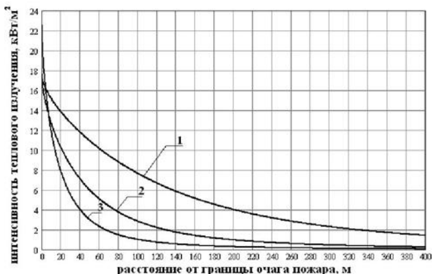
Рис. 3.2.5. Зависимости интенсивности теплового излучения от расстояния до границы очага пожара, при площади очага:
