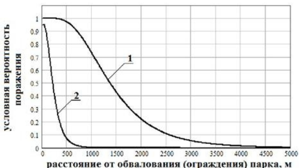
Рис. 3.2.11. Зависимости условных вероятностей поражения человека волной давления от расстояния до обвалования (ограждения) парка Q_{авт} - кривая 1, Q_{авт} - кривая 2
