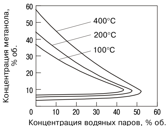
РИС. М.3. Концентрационные пределы распространения пламени смеси метанол – водяной пар – воздух при 100, 200 и 400^\circ\text{C} (давление атмосферное, МВСК 9,4\% об.; разбавление водяным паром при 120^\circ\text{C} )
