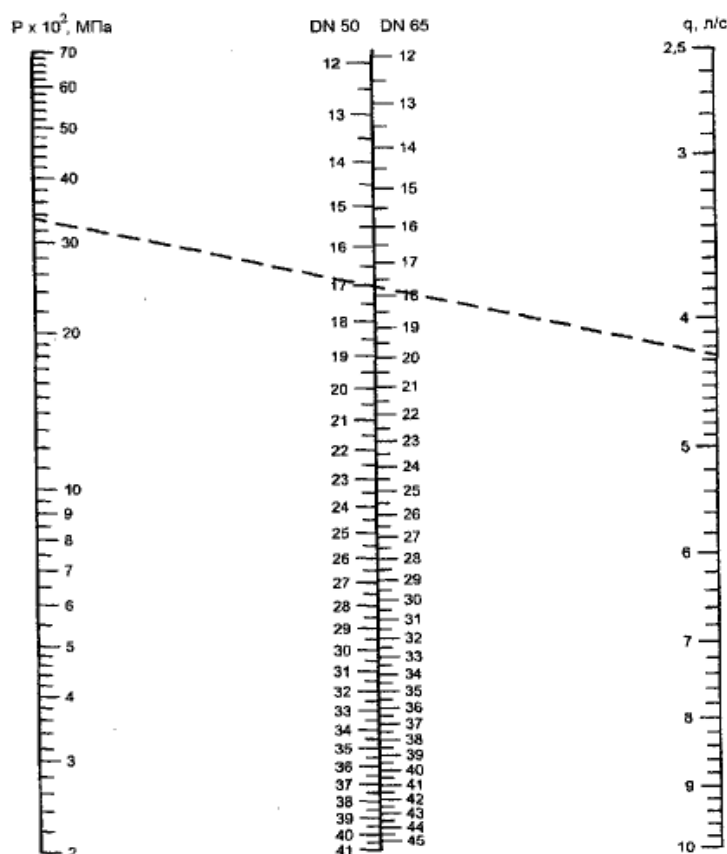
Номограмма для определения диаметра отверстия диафрагмы
