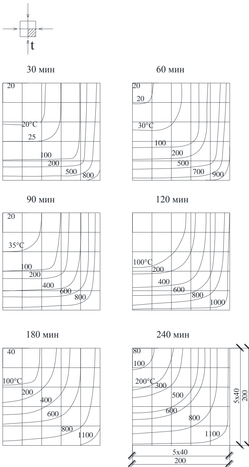
Рисунок И.9 - Балка из легкого бетона сечением 320х160 мм при нагреве с трех сторон
